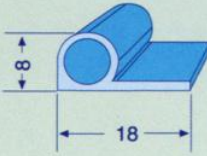
ER196 KAPAK LASTİĞİ
