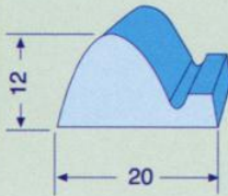
ER211 KAPAK CONTASI
