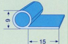
ER199 KAPAK LASTİĞİ
