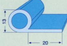
ER197 RAMÖZ KAPAK LASTİĞİ
