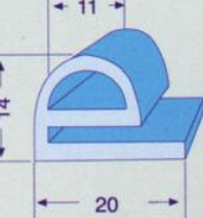
ER187 KAPAK LASTİĞİ
