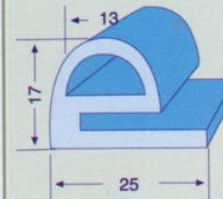
ER185 KAPAK LASTİĞİ
