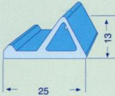
ER197 RAMÖZ KAPAK LASTİĞİ
