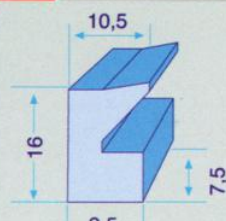
ER217 KAPAK LASTİĞİ
