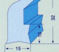
ER168 KEÇE LASTİĞİ
