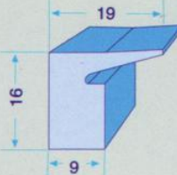
ER215 KAPAK LASTİĞİ
