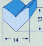
ER167 KAPAK LASTİĞİ
