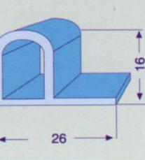
ER188 RAMÖZ KAPAK LASTİĞİ
