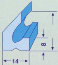
ER211 KAPAK CONTASI
