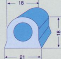
ER188 RAMÖZ KAPAK LASTİĞİ
