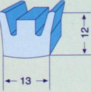
ER177 KAPAK LASTİĞİ
