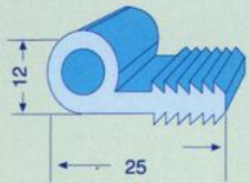
ER200 CONTA LASTİĞİ
