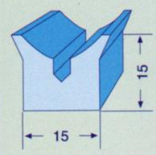
ER171 RAMÖZ KAPAK LASTİĞİ
