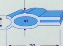
ER183 KAPAK LASTİĞİ
