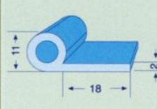
ER198 KAPAK CONTASI
