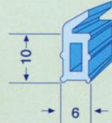
ER208 KARE SİLİKON LAMA
