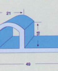
ER187 KAPAK LASTİĞİ
